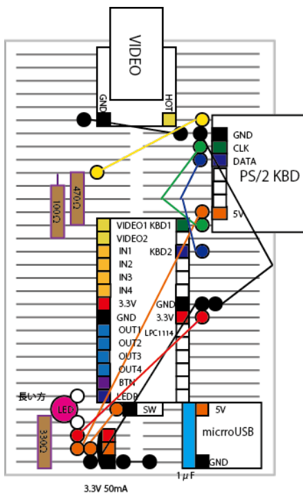
IchigoJam ver0.8.8 / 2014.11.28
